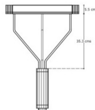
ALZADO
